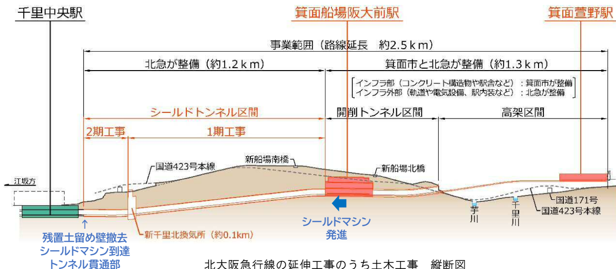
北大阪急行線の延伸工事のうち土木工事 縦断図 (千里中央駅～箕面船場阪大前駅間の残置土留め壁撤去、シールドトンネル工事)
