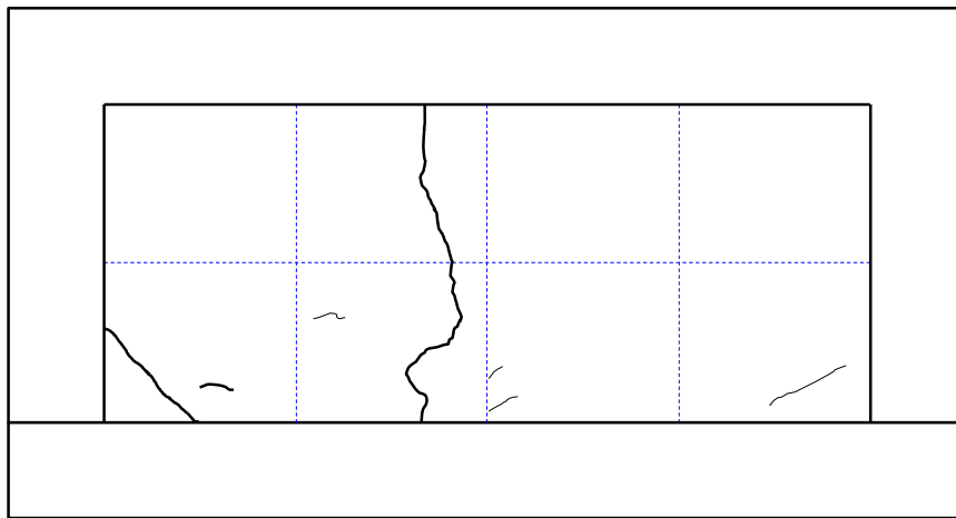
打設後 24 ヶ月の壁試験体の状況 【普通コンクリート（目標収縮ひずみ 800 \times 10^{-6} ）】
