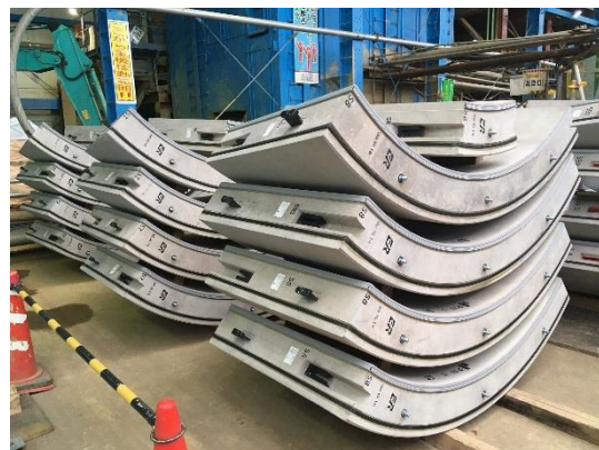
写真2 RCセグメント
