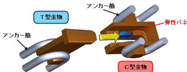
図1 FN継手の概要図
