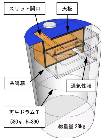
図1 円淵トンネルに設置した「ドラムサイレンサー」
