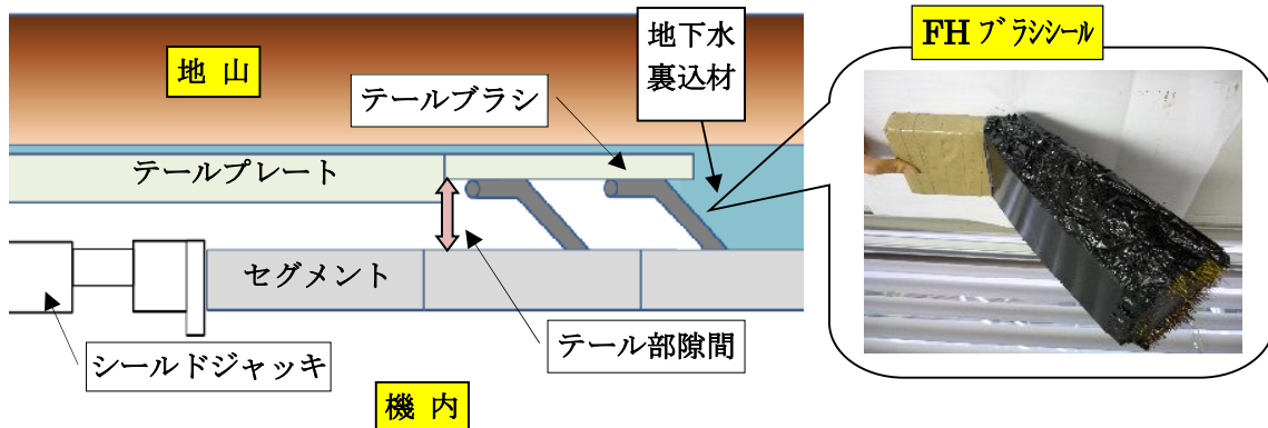
図1 シールドテール部イメージ
